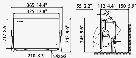
多功能显示器 (台式安装) TZTL12F 3.8 kg 8.4 lb
