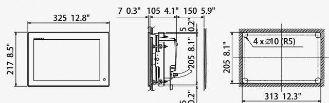
多功能显示器 (嵌入式安装) TZTL12F 3.7 kg 8.2 lb
