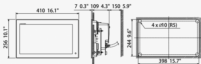
多功能显示器 (嵌入式安装) TZTL15F 4.8 kg 10.6 lb
