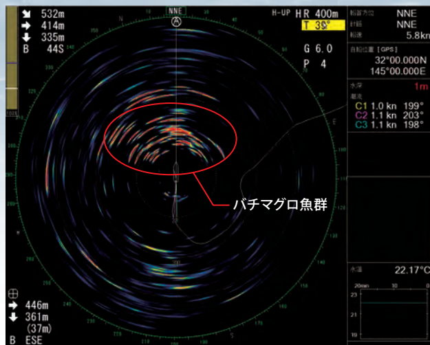
【400 mレンジ】バチマグロ魚群を単体魚に分離している。
