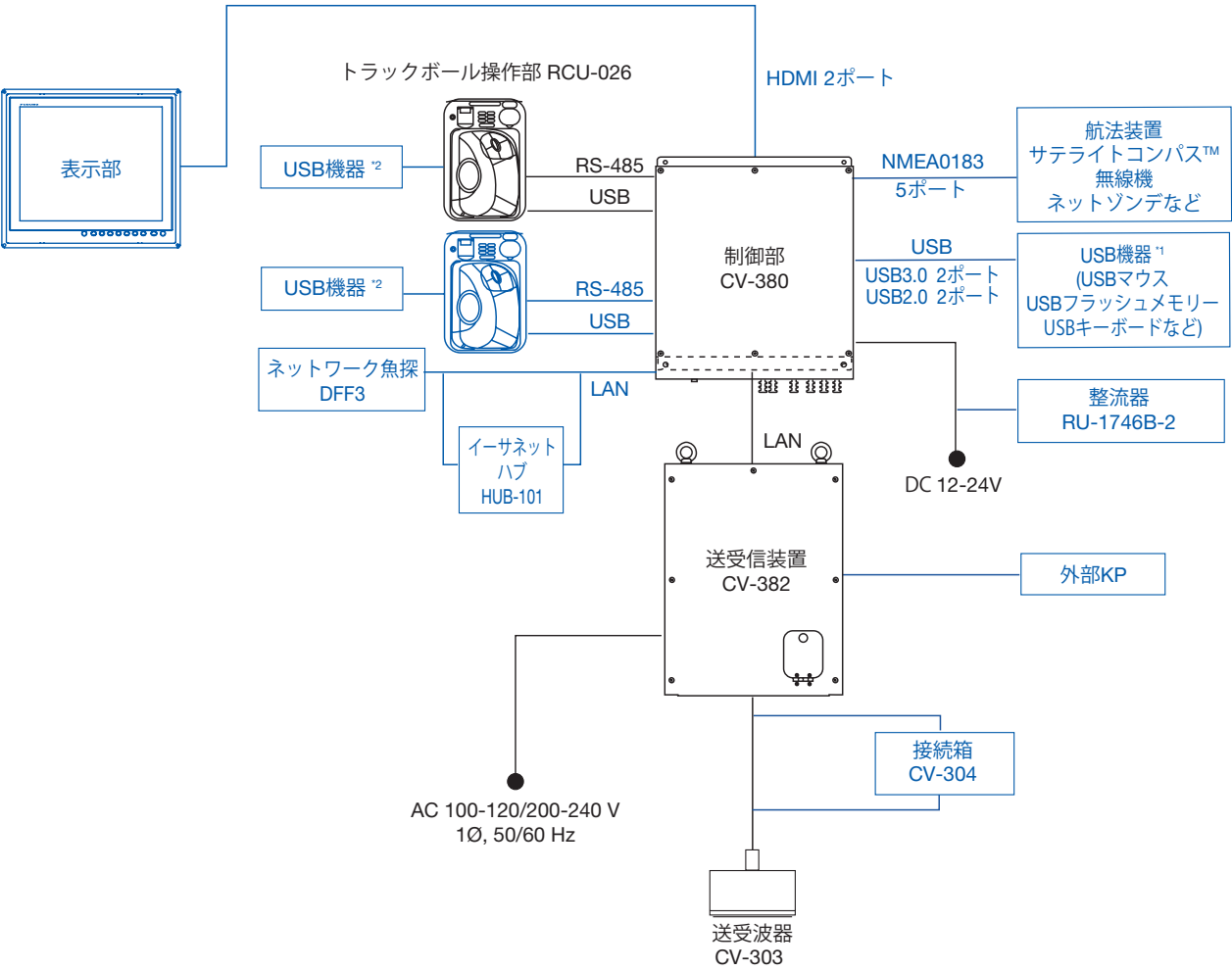
相互系統図
