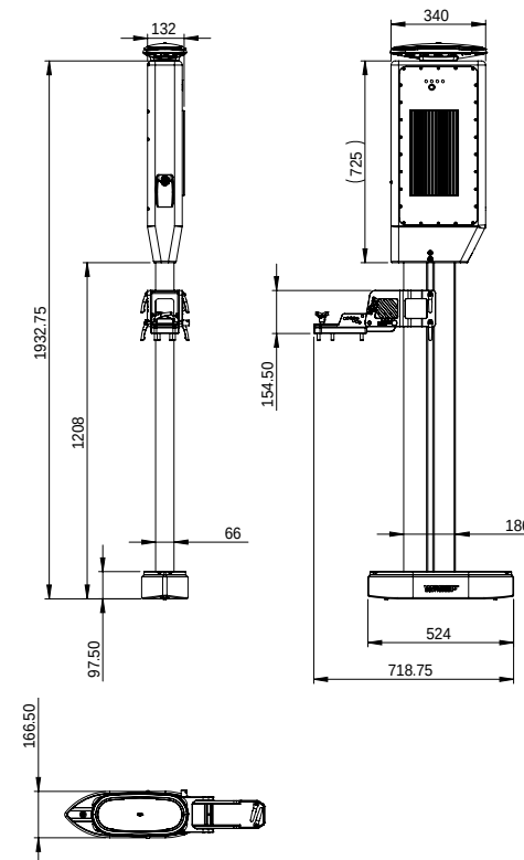
WMBW3P-160E Assembly
