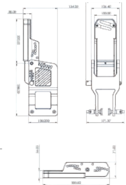
WMBW3P-160E Bracket
