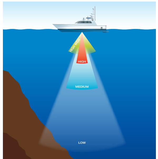
送受波器タイプごとの探知イメージ
