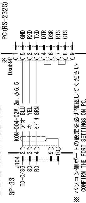
パソコン接続の例 EXAMPLE FOR PC CONNECTION
